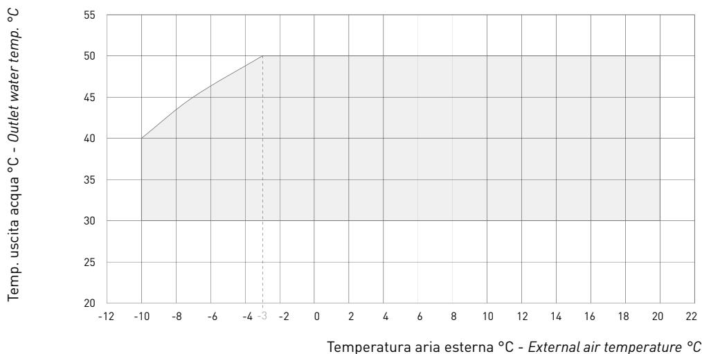
Fig.6: Limiti di funzionamento indicativi in modalità pompa di calore (HON). Indicative working limits in heat pump mode (HON).
