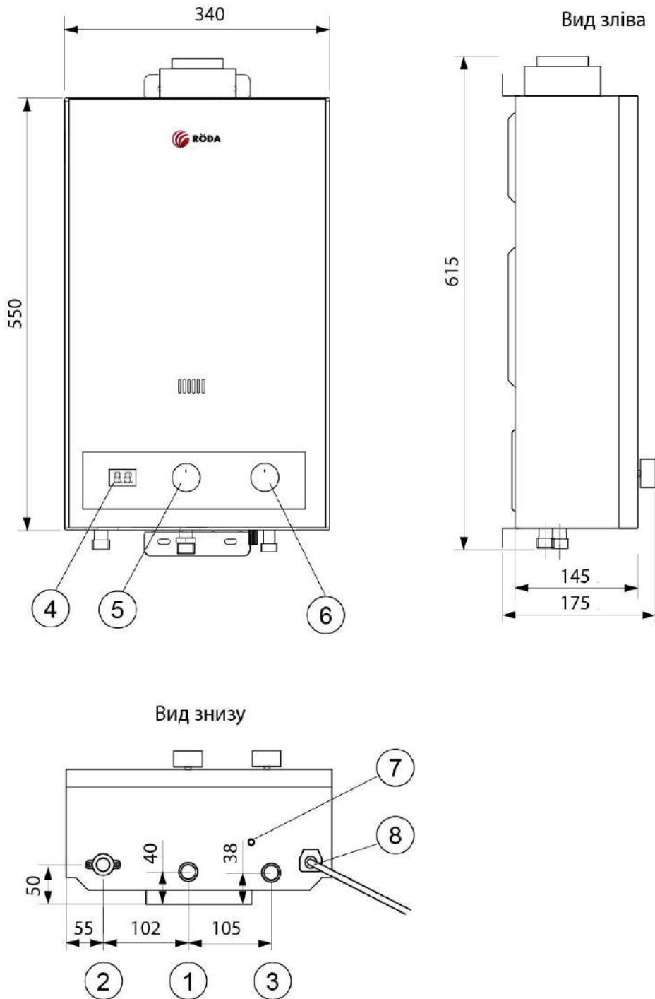
Рисунок 1. Розміри та основні елементи водонагрівача JSD-20T2M
