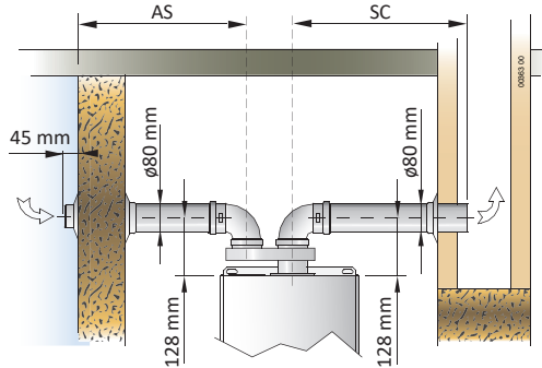
Приклад роздільної системи (C 32 )
