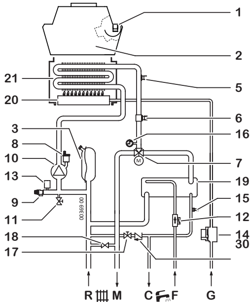
Модель Micra Duo OC (відкрита камера згоряння)
