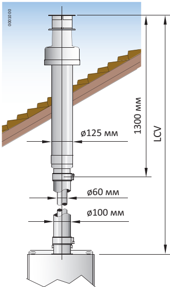
Приклад вертикальної коаксіальної системи (C 22 )
